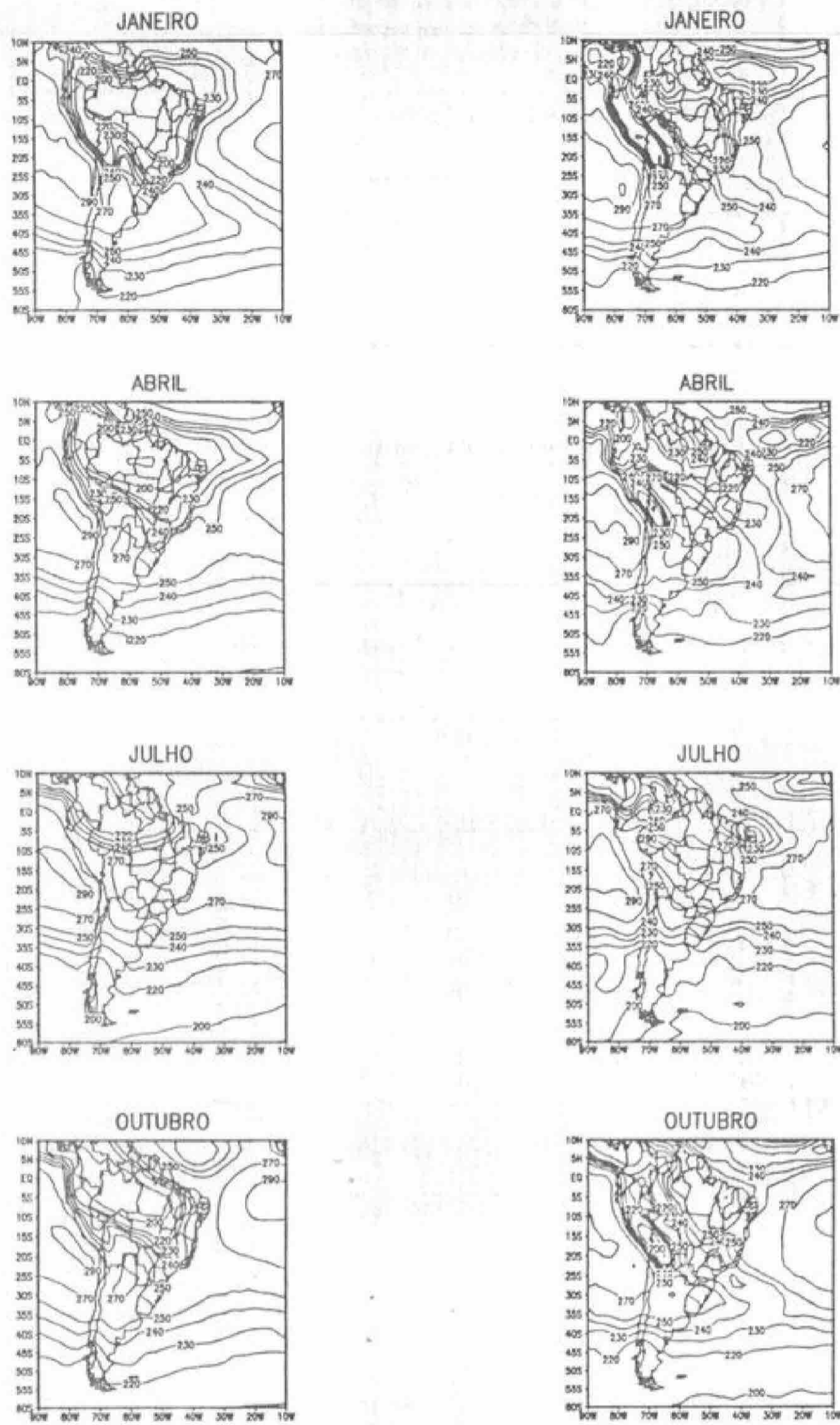
Figura 2. Radiação de Onda Longa (W/m 2 ) simulado pelo MCGA CPTEC /COLA coluna a direita comparada com a reanálise do NCEP coluna a esquerda.
