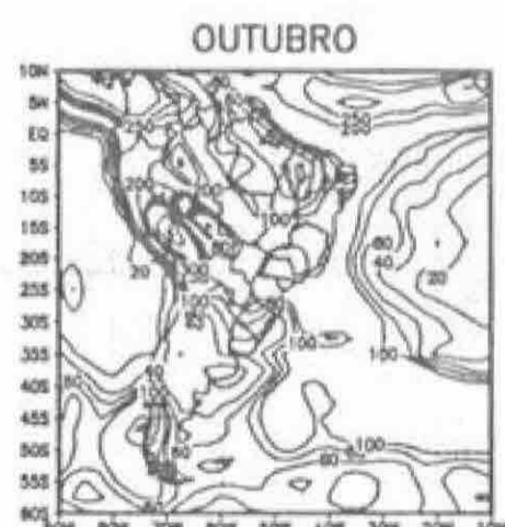
Figura 1. Precipitação total (mm/mês) simulada pelo MCGA CPTEC COLA, coluna a direita comparada com a reanálise do NCEP coluna a esquerda.
