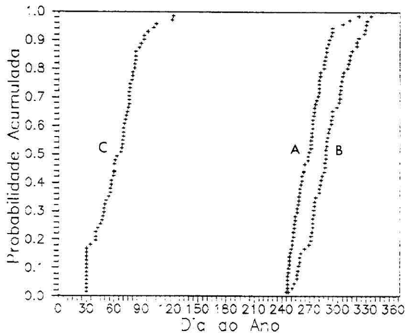
Fig. 3. Distribuições de probabilidade para o início efetivo (A), efetivo (B) e fim (C) da estação chuvosa.
