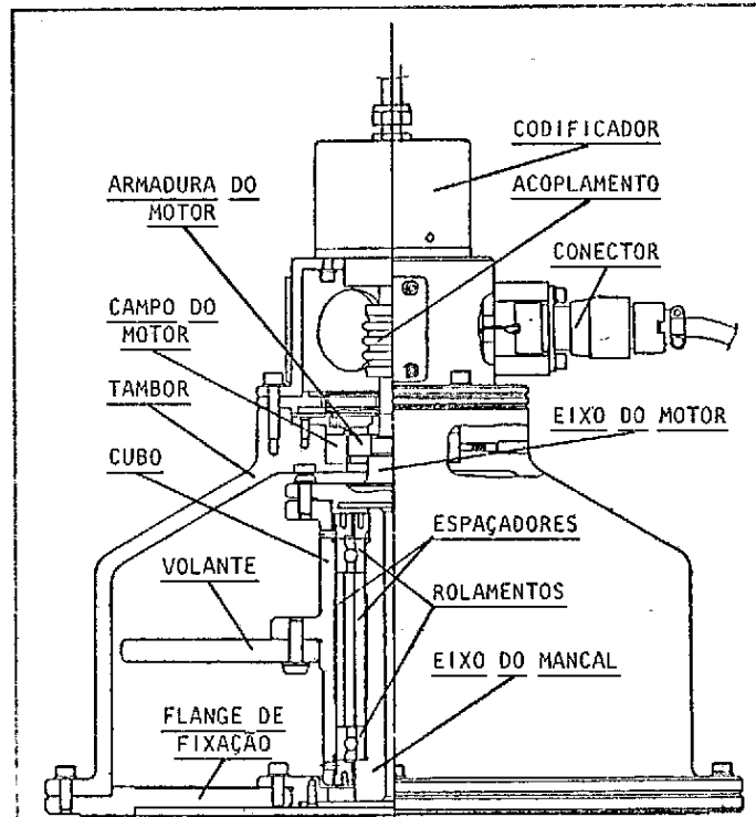
Fig. 1 - Vista em corte da roda de reação.
