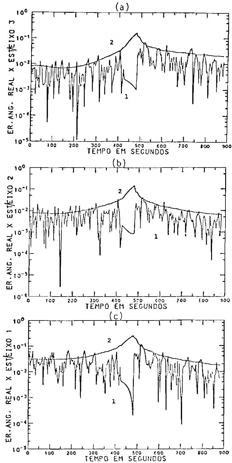
Fig.4.21 - Curvas sobrepostas dos erros angulares real ( \Delta\theta ) e estimado ( \hat{\delta}\theta ) (teste crítico). 1) erro real \Delta\theta ; 2) erro estimado \hat{\delta}\theta . a) eixo 3; b) eixo 2; c) eixo 1.
