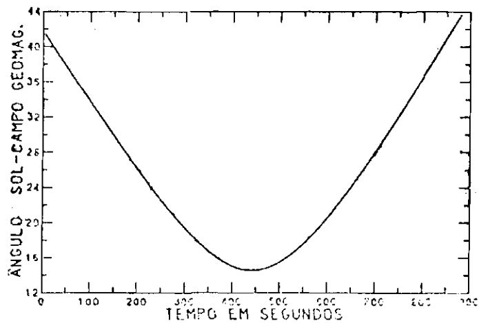
Fig. 4.11 - Ângulo \alpha entre a direção do Sol e do campo geomagnético visto do satélite (teste mediano).
