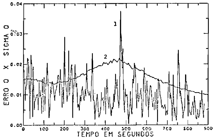
Fig. 4.13 - Curvas sobrepostas dos erros real ( \Delta q ) e estimado ( \delta q ) para a atitude (teste mediano). 1) erro real \Delta q ; 2) erro estimado \delta q .
