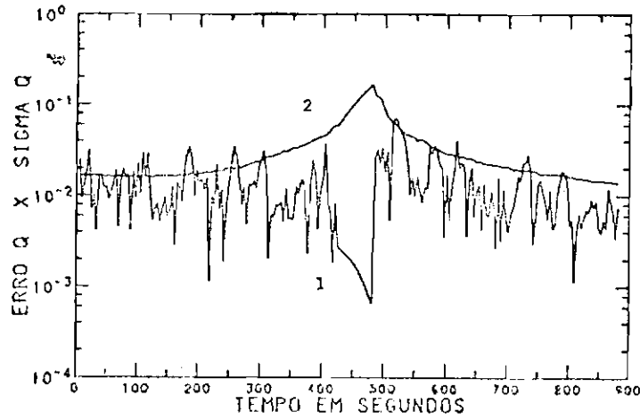
Fig. 4.19 - Curvas sobrepostas dos erros real ( \Delta q ) e estimado ( \delta q ) para a atitude (teste crítico). 1) erro real \Delta q ; 2) erro estimado \delta q .
