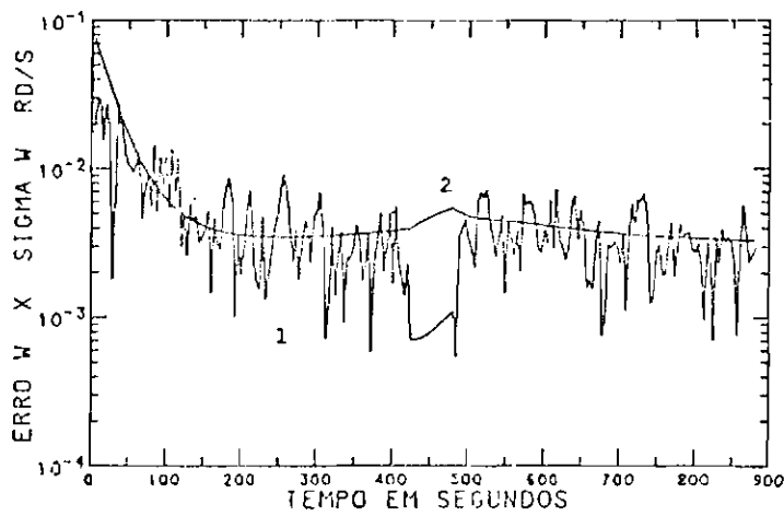
Fig. 4.20 - Curvas sobrepostas dos erros real ( \Delta \omega ) e estimado ( \delta \omega ) para a velocidade angular (teste crítico). 1) erro real \Delta \omega ; 2) erro estimado \delta \omega .
