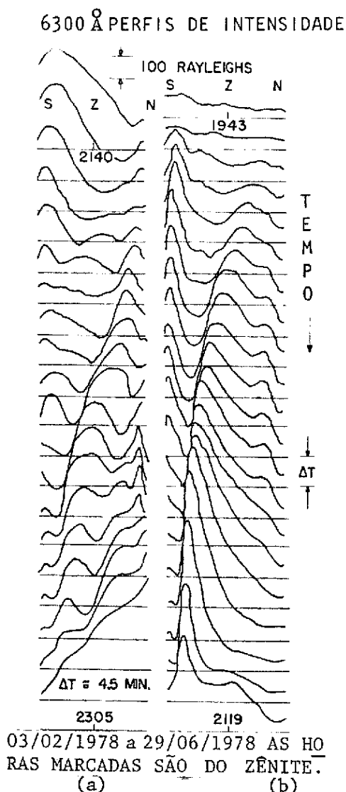
Fig. 1 - Perfis meridionais da luminescência noturna do oxigênio atômico, no comprimento de onda de 6300 Å.
