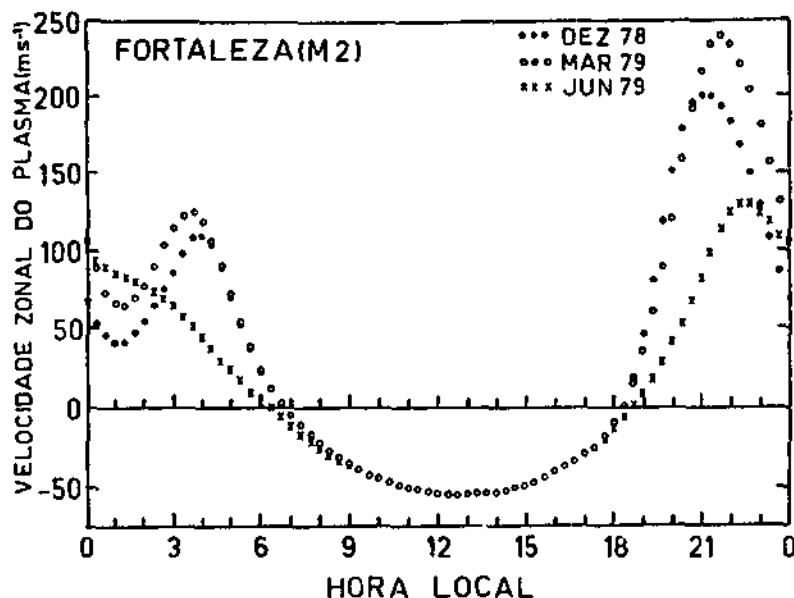
Figura 1 - Variação diurna da velocidade de deriva zonal do plasma da região F a 350 km de altura sobre Fortaleza, obtida usando o modelo M2 para os meses de dezembro de 1978 ( . . ), março de 1979 (o o o) e junho de 1979 (x x x).
