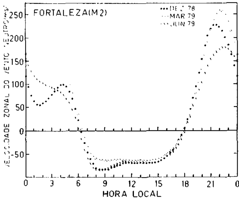
Figura 4 - Variação diurna da componente zonal do vento neutro termosférico a 350 km sobre Fortaleza, obtida usando o modelo M2 para dezembro de 1978 ( . . . ), março de 1979 (o o o) e junho de 1979 (x x x).
