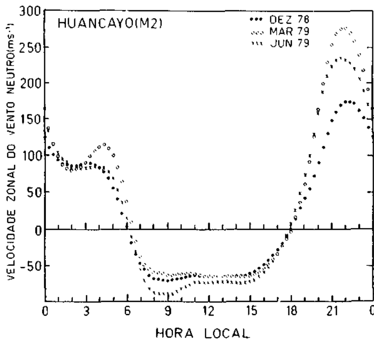
Figura 5 - Variação diurna da componente zonal do vento neutro termosférico a 350 km sobre Huancayo, obtida usando o modelo M2 para dezembro de 1978 ( . . . ), março de 1979 (o o o) e junho de 1979 (x x x).
