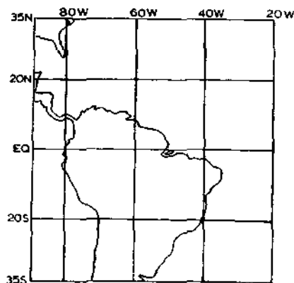
Fig. 1. Região para o estudo da simulação em projeção mercator
