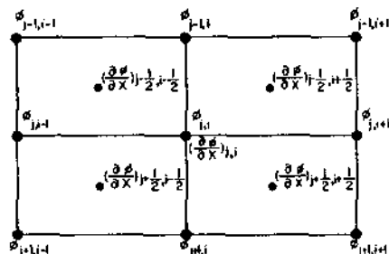
Fig. 3. Os nove pontos utilizados no esquema de diferenças finitas no espaço (semi-momentum de Schuman)
