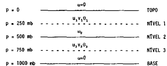
Fig. 2. Distribuição das variáveis nos vários níveis no modelo utilizado, onde estão indicados os níveis de pressão. O topo é tomado em p = 0 \text{ mb} . Nos níveis 1 e 3, tem-se os campos de vento e da temperatura potencial. No nível 2, no topo e na base estão indicadas as velocidades verticais
