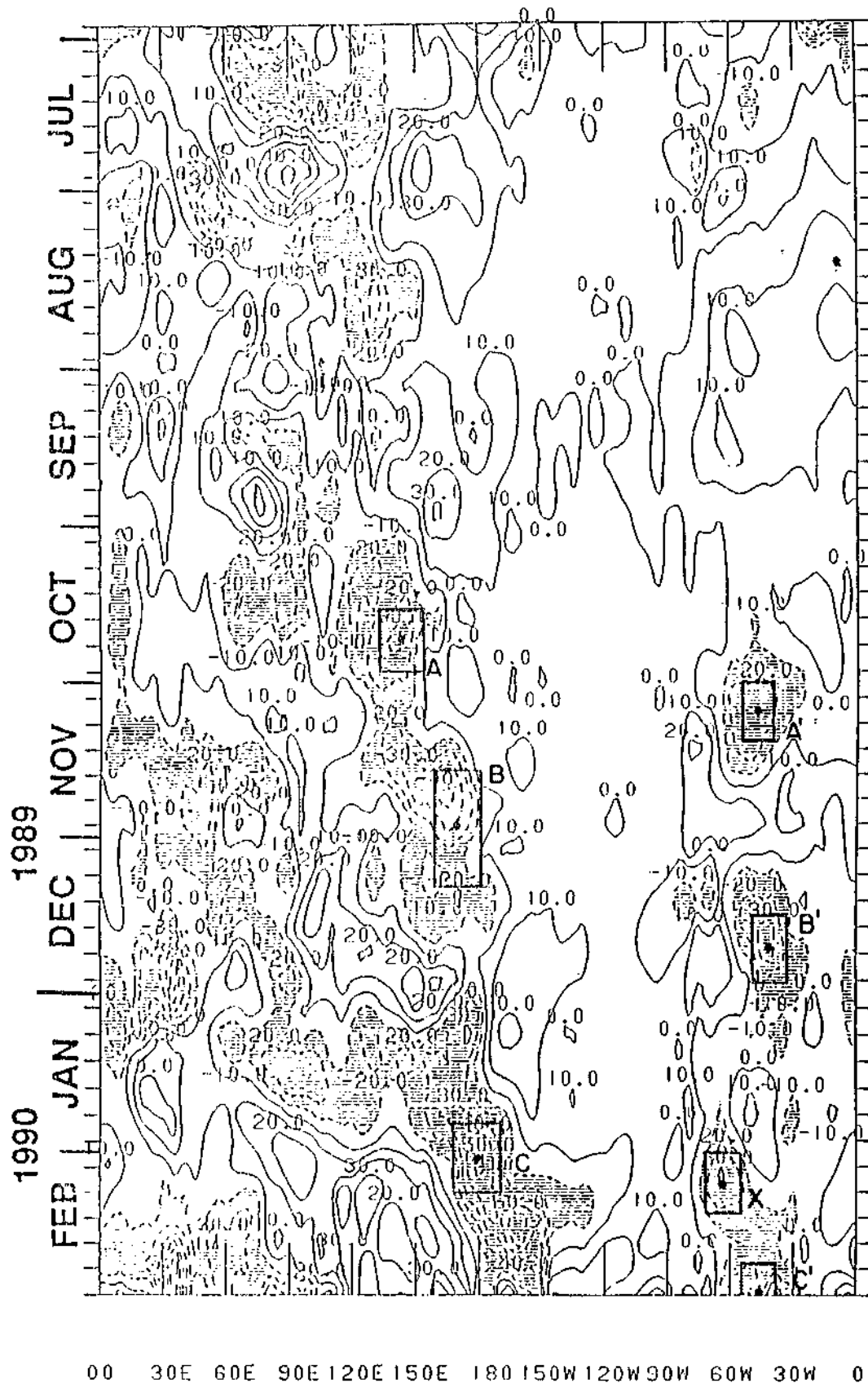
FIG 1 - Seção tempo versus longitude de anomalias de radiação de onda longa para a faixa 5^{\circ}\text{N} - 5^{\circ}\text{S} . As anomalias foram computadas para cada pântada. O intervalo é 10\text{ W/m}^2 . Isolinhas de valores positivos (negativos) estão representadas por linhas cheias (tracejadas). Valores inferiores a -10\text{ W/m}^2 estão hachuradas. (LONIE: Climate Diagnostics Bulletin, 1990).
