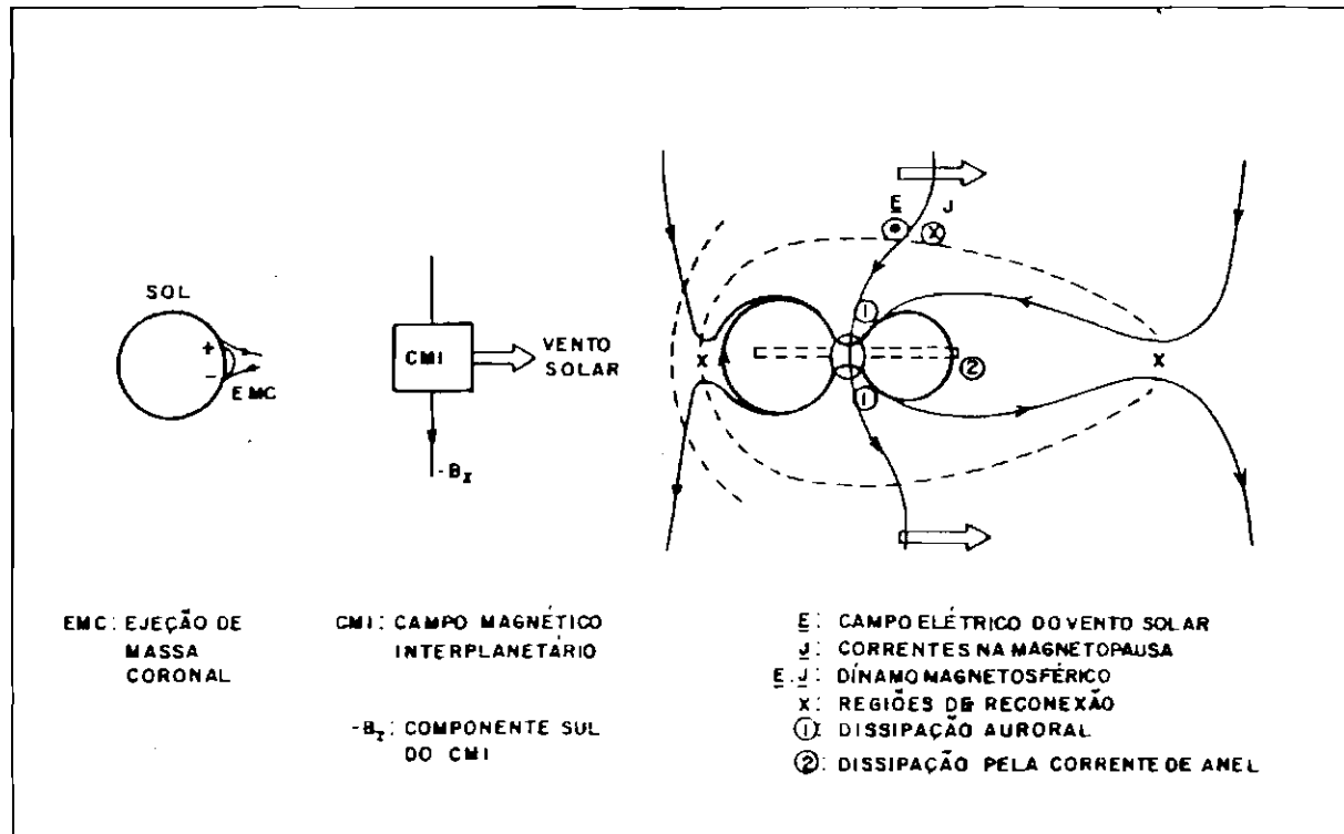
Fig. 2.9 - Esquema do acoplamento sol-magnetosfera. FONTE: Gonzalez et al. (1992), p. 12.
