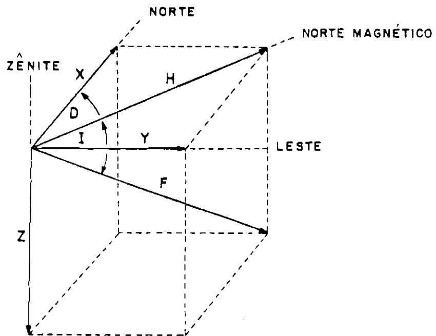
Fig. 1.1 - Componentes do vetor do campo geomagnético
