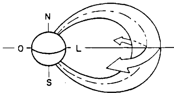
Fig. 2.3 - Corrente de anel. FONTE: Papagiannis (1983), p. 167.
