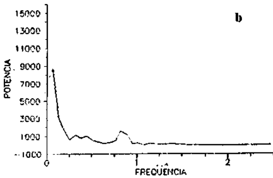
Fig. 3 - Espectro de potência para as pentadas móveis da precipitação sobre a região do Cariri para novembro a maio de: a) - o), para 1974/75 a 1988/89, respectivamente. A unidade das ordenadas é \text{mm}^2 \text{dia}^{-1} e a das abscissas é \text{dia}^{-1} .
