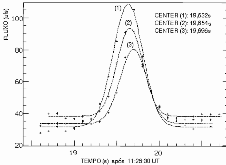
Fig. 3.5 - Deslocamento do t_m , mostrando a taxa de deriva em frequência de uma explosão tipo III, observada em 05-set-92. Os perfis temporais correspondem às frequências de 594 MHz (1), 580 MHz (2) e 566 MHz (3).
