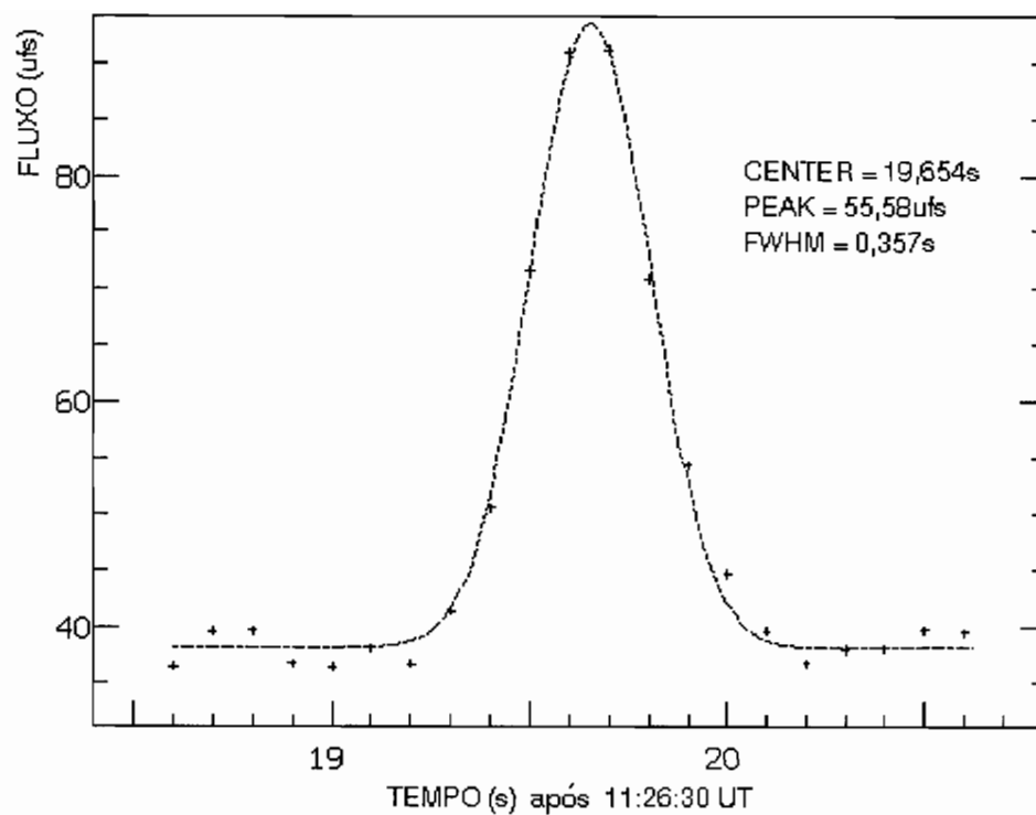
Fig. 3.2 - Ajuste gaussiano ao perfil temporal de uma explosão tipo III na frequência de 580 MHz observada no dia 05-set-92 (Tarefa imexamine do IRAF).
