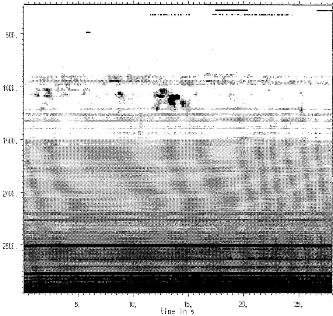
Fig. 2.4 - Espectro dinâmico de explosões solares decimétricas tipo “patch” observadas em 07/set/92 (07:11:13 UT) pelo Rádio Espectrômetro PHOENIX. O eixo vertical corresponde à frequência em MHz.
