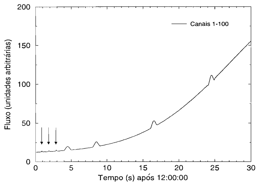
Fig. 5.3 - Perfil temporal integrado em todos os canais, das explosões da Figura anterior. As primeiras três explosões tipo “spikes”, são assinaladas com setas.
