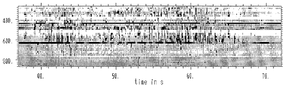
Fig. 2.3 - Espectro dinâmico de explosões solares decimétricas tipo “spike” observadas em 03/out/93 pelo Rádio Espectrômetro PHOENIX. O eixo vertical corresponde à frequência em MHz.
