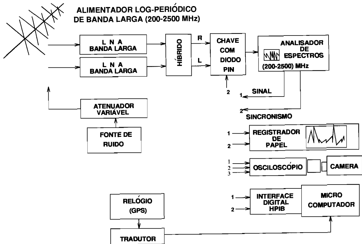
Fig. 5.1 - Diagrama de blocos representando o Espectrógrafo Decimétrico Digital de Banda Larga com alta sensibilidade e altas resoluções temporal e espectral (WDDHRS). Fonte: Adaptada de Sawant et al. (1996), p. 386.
