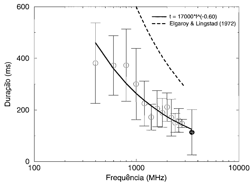
Fig. 3.7 - Duração das explosões tipo III decimétricas. O círculo preto corresponde às medições de Stahli e Benz (1987) para 3500 MHz, e a linha tracejada é a extrapolação para a faixa decimétrica da relação empírica de Elgaroy e Lingstad (1972).
