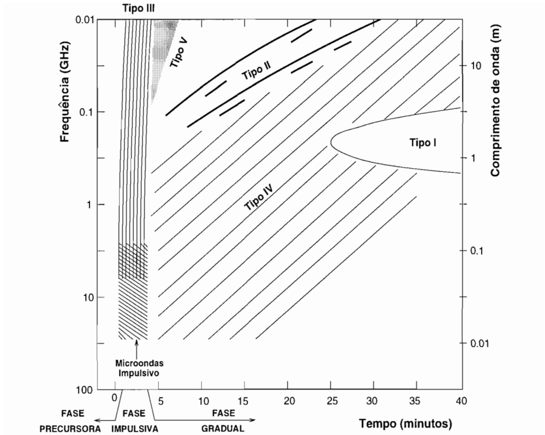
Fig. 1.2 - Representação dos diferentes tipos de explosões solares observadas na faixa de rádio frequências (10 – 30000 MHz). FONTE: Adaptada de Dulk (1985), p. 169, e atualizada incluindo as várias fases do “flare”, e as recentemente observadas explosões tipo III até 6 GHz.
