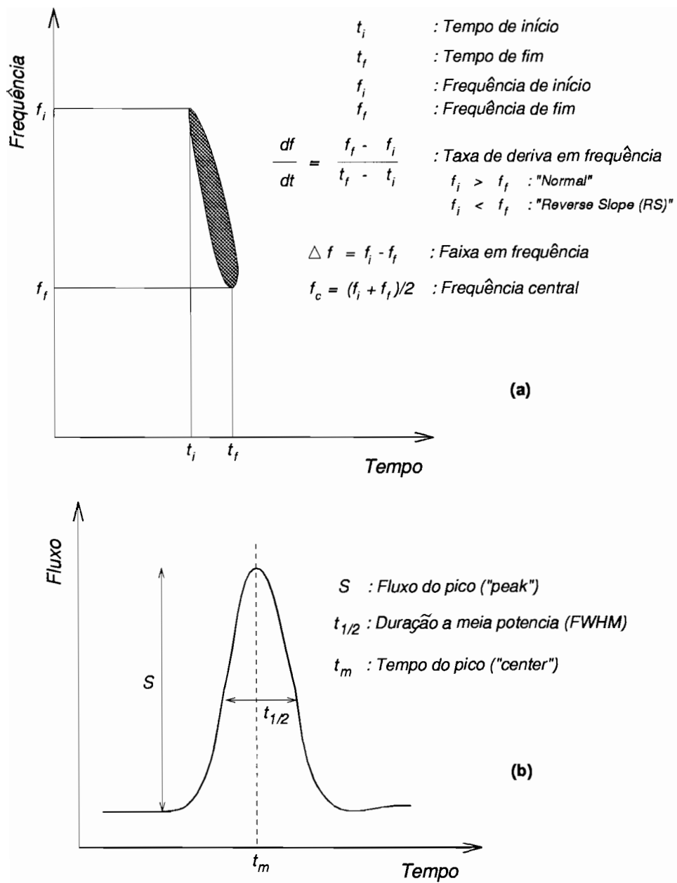
Fig. 3.1 - Esquema com os diferentes parâmetros de uma explosão tipo III. (a) Espectro dinâmico e (b) perfil temporal em uma dada frequência.
