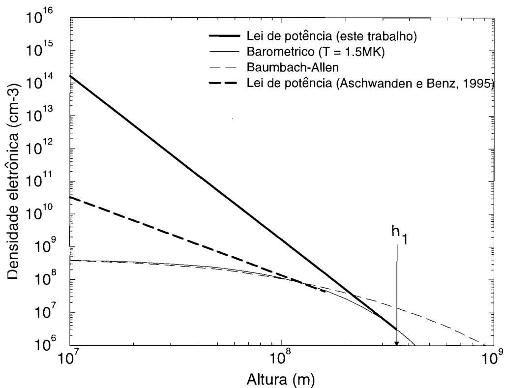
Fig. 4.1 - Modelo de densidade para “loops” emissores de explosões tipo III. O modelo de lei de potência para a baixa coroa ( h < h_1 ) é mostrado pela linha contínua-grossa (este trabalho), junto ao modelo de Aschwanden e Benz (1995) mostrado pela linha tracejada-grossa. A linha fina mostra a componente barométrica para a coroa superior ( h > h_1 ). O modelo de Baumbach-Allen (linha fina-tracejada) é mostrado para comparação.
