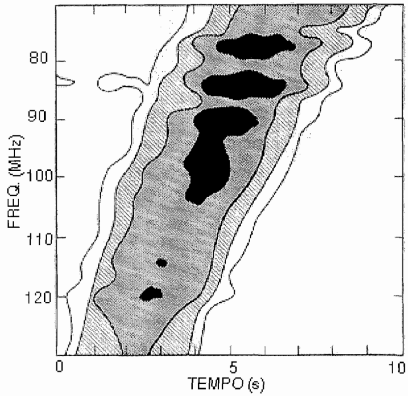
Fig. 1.4 - Espectro dinâmico de uma explosão tipo III. O eixo horizontal representa o tempo em segundos, e o eixo vertical a frequência em MHz. Os registros mais escuros indicam maior fluxo. FONTE: Wild e McCready (1950), p. 387.
