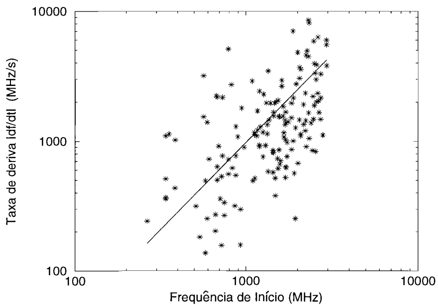
Fig. 3.11 - Ajuste dos valores absolutos das taxas de deriva ( df/dt ).
