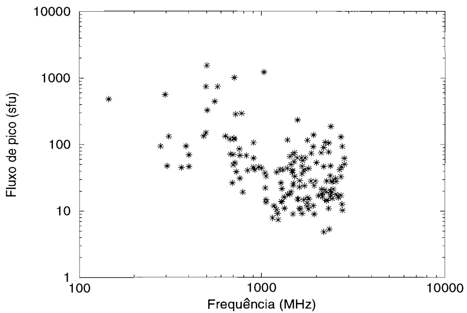
Fig. 3.13 - Gráfico de fluxo de pico vs frequência das explosões tipo III decimétricas.
