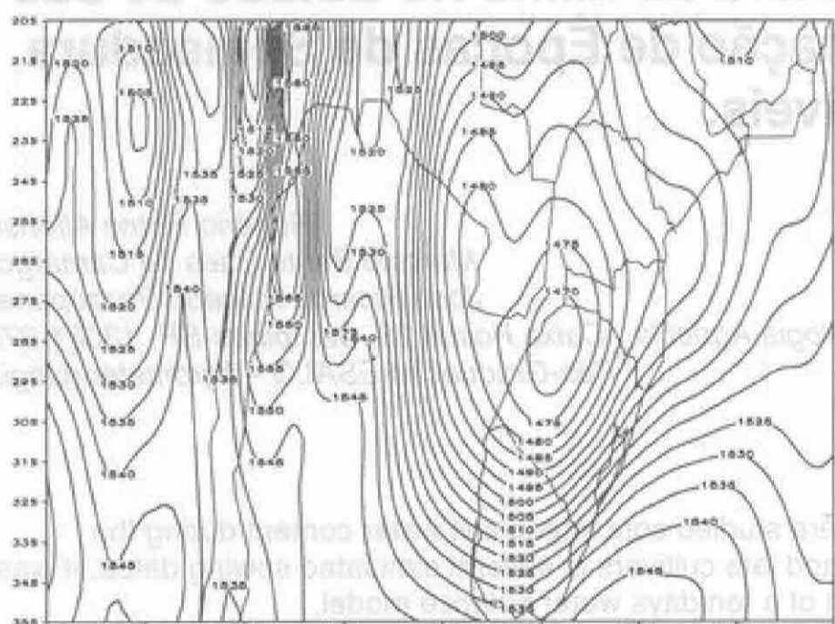
Figura 3.a: Campo de altura geopotencial [m] para os dias 24, no nível de 850 hPa
