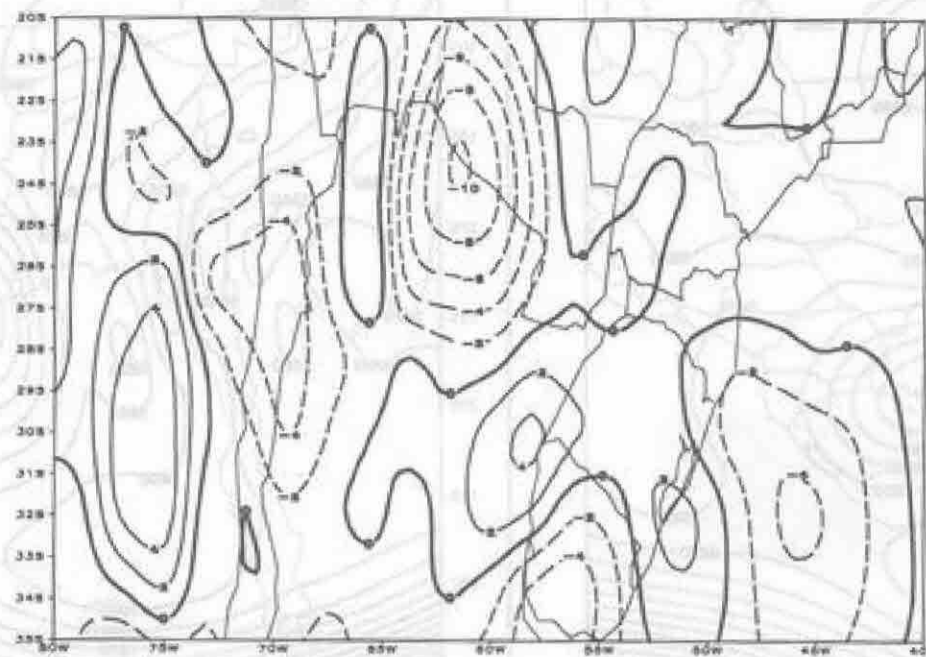
Figura 6: campo de advecção de temperatura [ ^{\circ}C \times s^{-1} ], no nível de 850 hPa, para o dia 24/12/1995.
