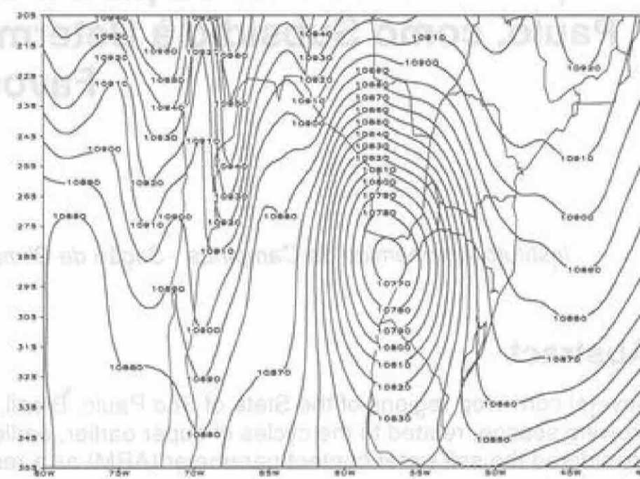
Figura 3.b: Campo de altura geopotencial [m] para os dias 24, no nível de 250 hPa
