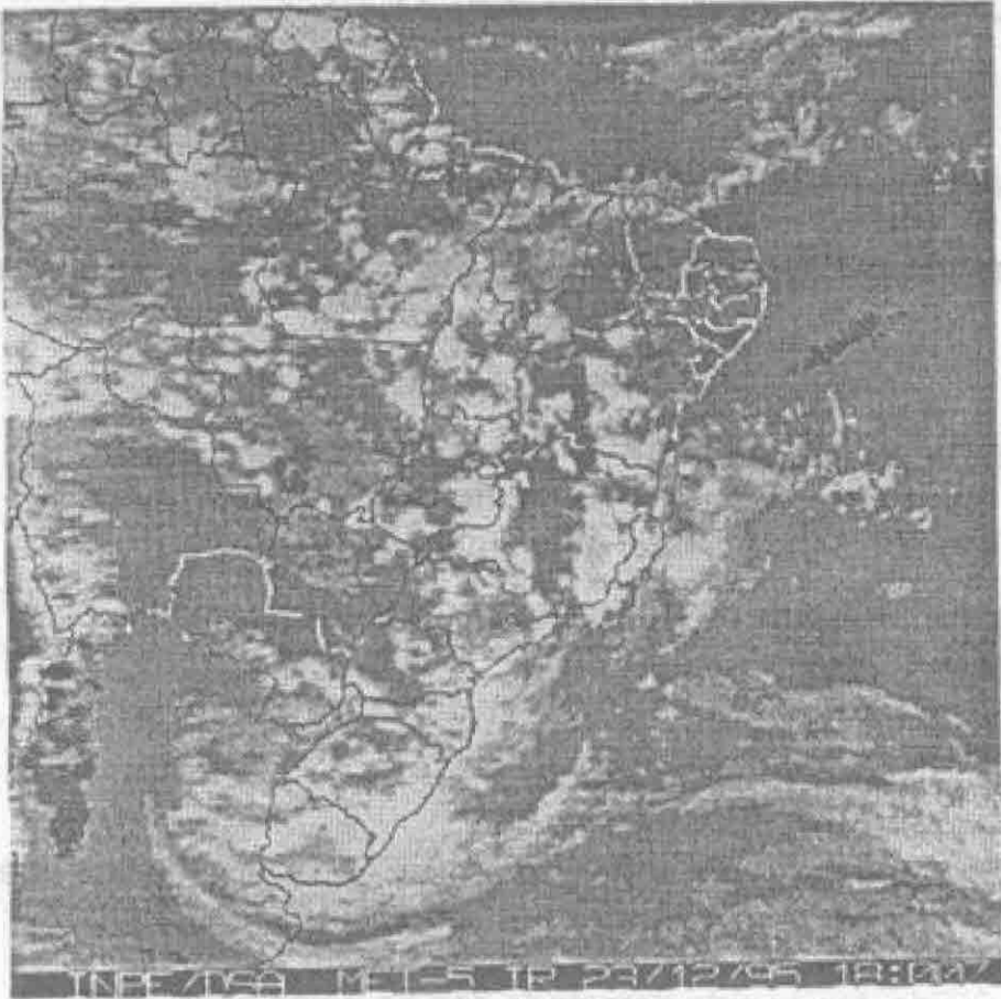
Figura 1.a: Imagem do satélite METEOSAT-5 para o dia 23/12/1995 às 18 UTC
