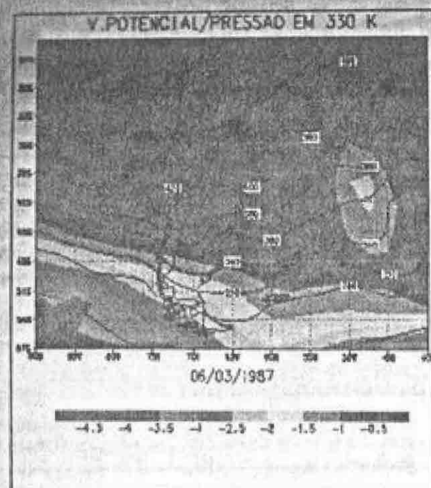
Fig.5- Campo de Vorticidade Potencial, para o dia 06 de março de 1987, na superfície isentrópica de 330 K.
