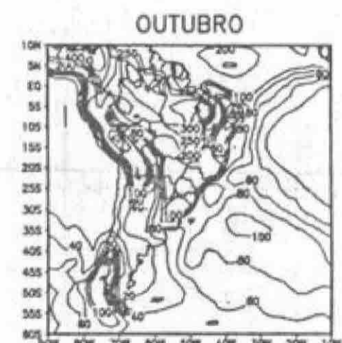
Figura 1. Precipitação total (mm/mês) simulada pelo MCGA CPTEC COLA, coluna a direita comparada com a reanálise do NCEP coluna a esquerda.
