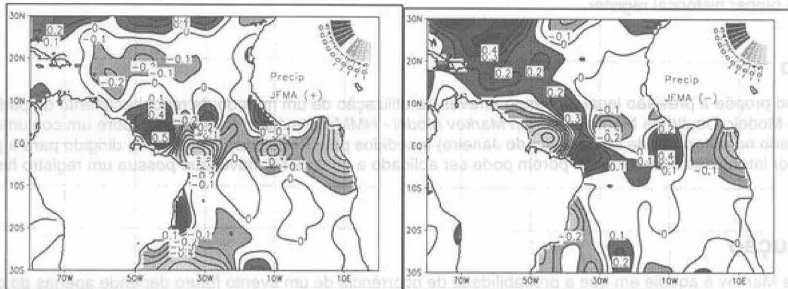
Fig. 6 -O mesmo que a Fig. 2, porém, para as anomalias de precipitação (mm).
