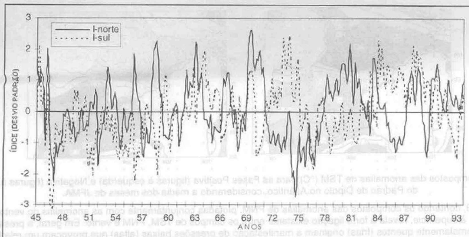
Fig. 1 -Série temporal dos índices normalizados médios mensais de TSM para as áreas ao norte (linha sólida) e ao sul (linha pontilhada) do equador sobre o Atlântico tropical.
