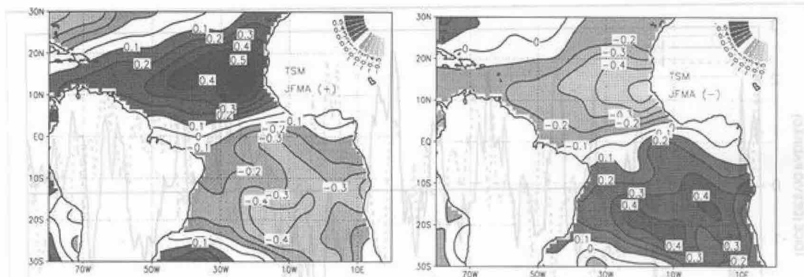
Fig. 2 - Compostos das anomalias de TSM (°C) para as Fases Positiva (figuras à esquerda) e Negativa (figuras à direita) do Padrão de Dipolo no Atlântico, considerando a média dos meses de JFMA.
