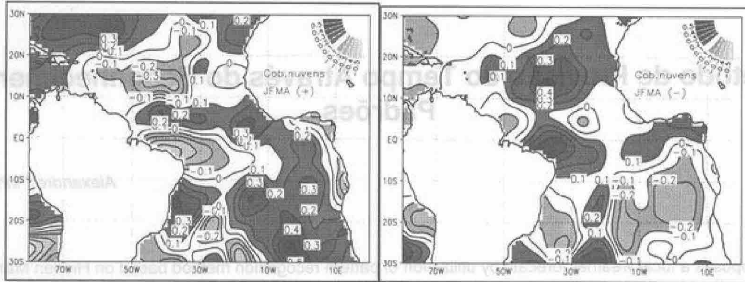
Fig. 5 -O mesmo que a Fig. 2, porém, para as anomalias de cobertura fracional de nuvens (%).
