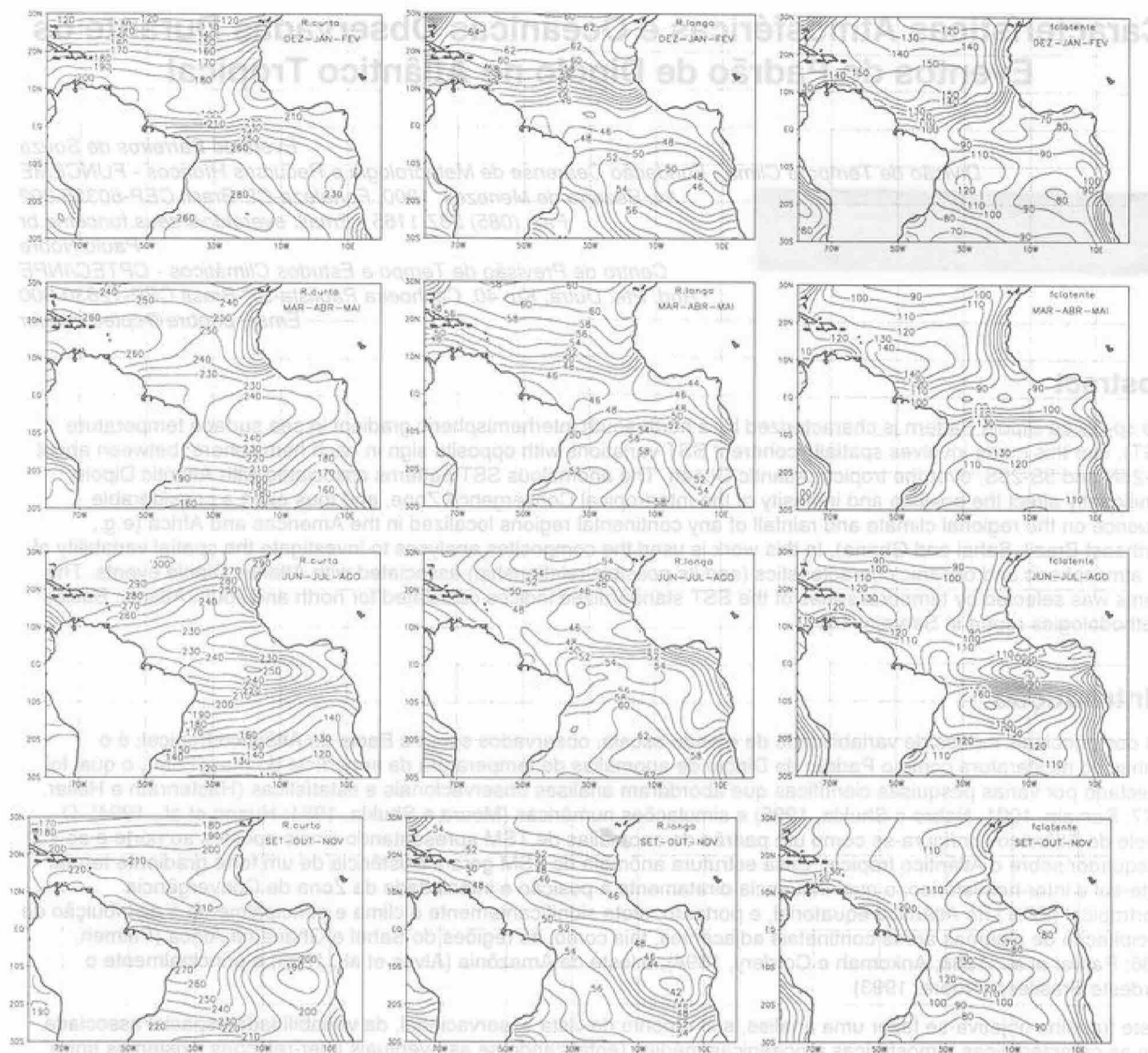
Fig. 3 - Médias climatológicas sazonais para os campos de radiações de ondas curtas ( W/m^2 ) (mapas à esquerda), ondas longas ( W/m^2 ) (mapas no centro) e fluxo de calor latente ( W/m^2 ) sobre o Atlântico Tropical, representativas aos meses de DJF, MAM, JJA e SON.
