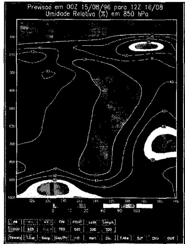
Fig. 3 - Corte vertical da umidade relativa.
