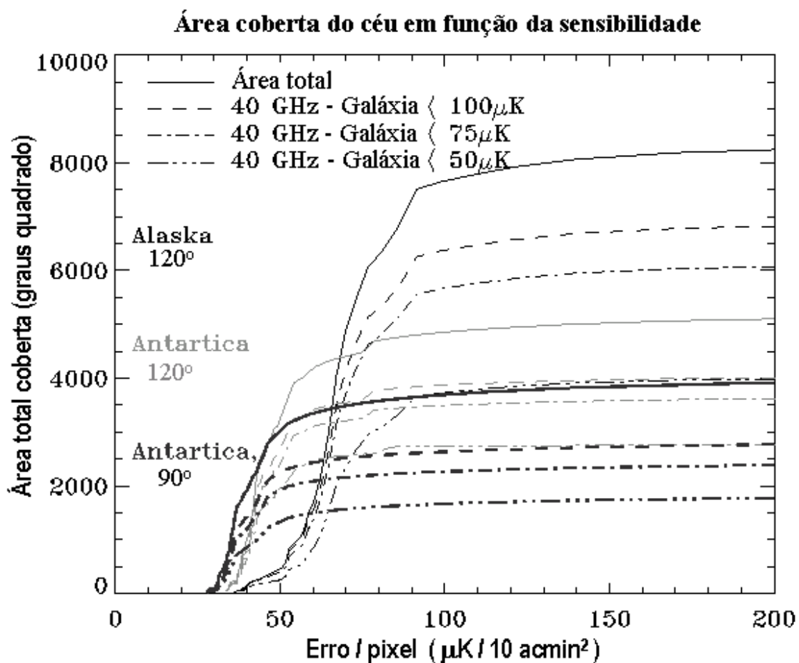
Figura 4.6 - Área total coberta em função da sensibilidade, com diferentes sensibilidades para diferentes cortes no Plano Galáctico. Foram consideradas apenas seis cornetas com uma sensibilidade de 300 \mu\text{K} \sqrt{s} .
