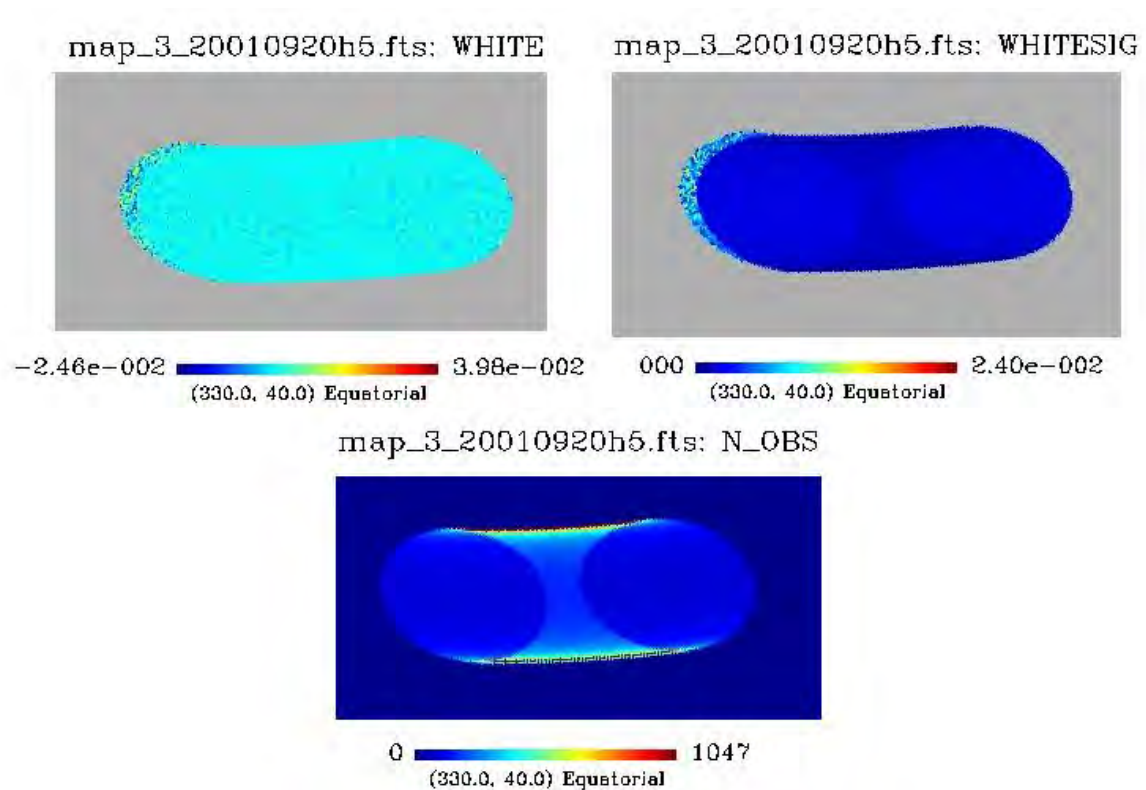
Figura 5.20 - Mapas em coordenadas gnomônicas do sinal (White), do ruído (Whitesig) e do número de vezes que cada pixel foi observado ( n_{obs} ) durante a terceira hora de observação realizada no dia 20/09/2001. O nome dos mapas é determinado pelo canal (3), pela data (20010920) na pela hora UT na qual os dados foram coletados (h5). No caso acima.
