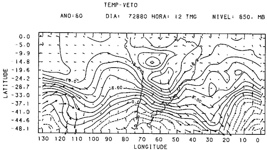
b) Escoamento e isotermas em 850mb.
