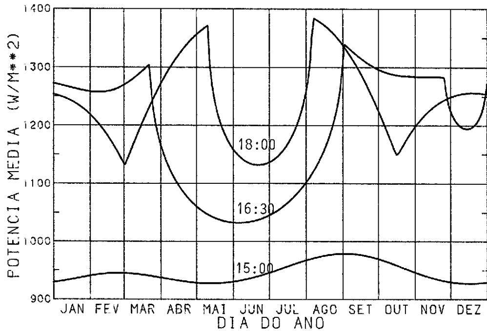
Fig. 4.6 - Potência média numa órbita, disponível nos painéis ao longo de um ano, para 3 horários de cruzamento distintos: \bar{h} = 15:00 h, 16:30 h e 18:00 h.
