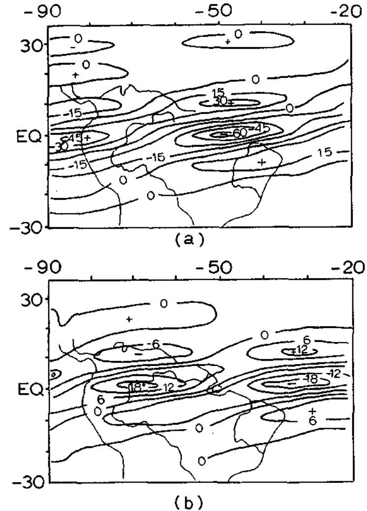
Fig. 6. Campo da velocidade vertical no nível de 500mb em unidades de 10^{-4} mb/s a) caso seco, b) caso chuvoso. Calculada 4 dias após o instante inicial. Nota-se no caso seco, que o movimento vertical é quase predominantemente descendente na região em questão.
