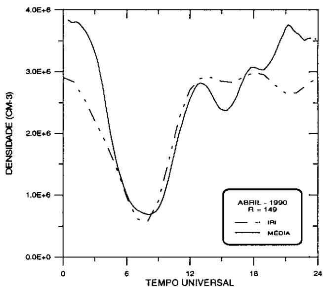
Fig.3.4 Média da variação diurna da densidade eletrônica do pico da camada F.
