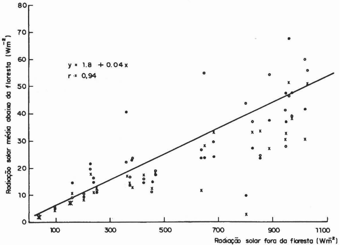
Fig. 2. Relação entre o fluxo de radiação solar incidente na clareira e o fluxo médio para 3 pontos amostrais no chão da floresta amazônica em Tucuruí, Pará. A reta é a melhor aproximação encontrada por mínimos quadrados entre a radiação solar média, alcançando o chão da floresta, e a radiação solar fora da floresta.
