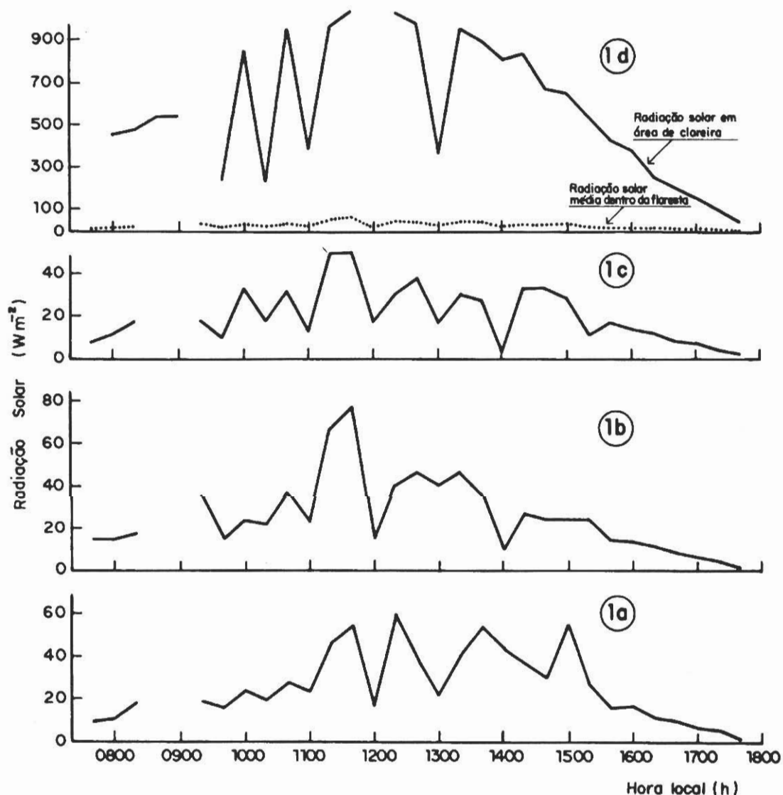
Fig. 1. Distribuição da radiação solar em função da hora local para 3 piranômetros instalados dentro da floresta (1a, 1b, 1c) e um situado em área aberta (1d). A radiação média para os 3 sensores da mata é apresentado em 1d. Medidas feitas em 07.11.86 em Tucuruí/PA.
